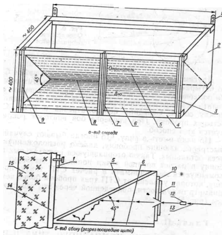
Рис. 1. Двухщитовой пулеулавливатель для стрельбы из пневматических винтовок:
